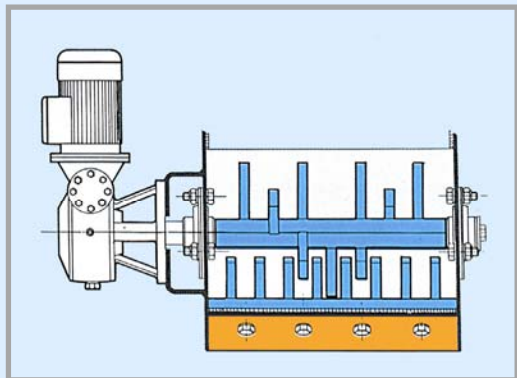
Prerompitore/alimentatore per prodotti non granulari. Pre-breaker/feeder for non granular products. Pré-briseur/alimentateur pour produits non granulaires.
