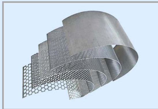
Vagli di perfetta tenuta con forature a richiesta. Airtight screens with various holes on request. Tenue étanche des grilles avec trous sur demande.
