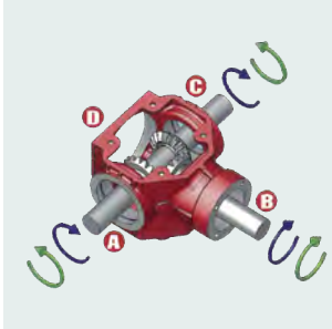
Moltiplicatore reversibile. Reversible gearbox.
